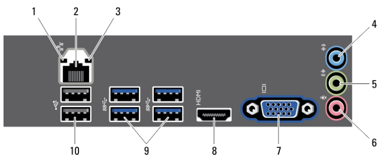
Skica 2. Pogled od zadaj
